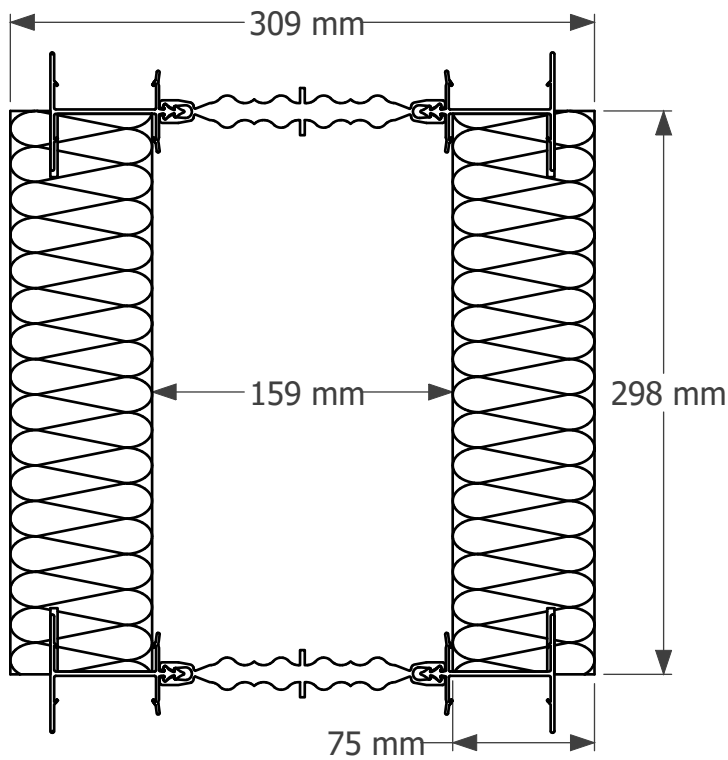
SCALE 1 : 4
